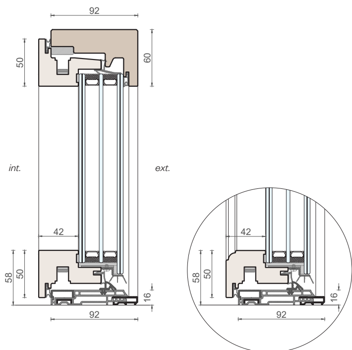
Sezione verticale
