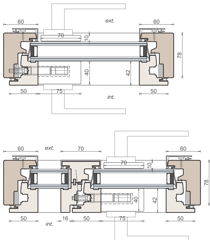
Sezione verticale
