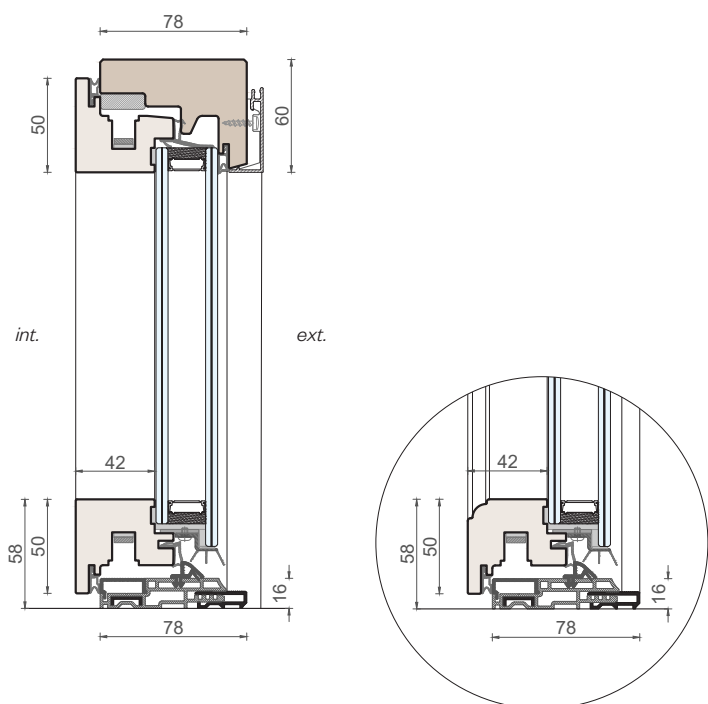
Sezione verticale
