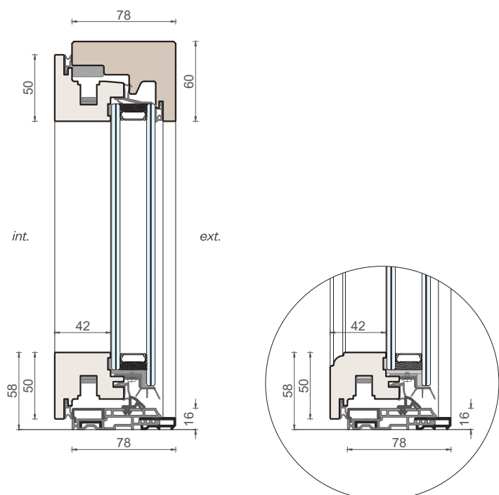
Sezione verticale
