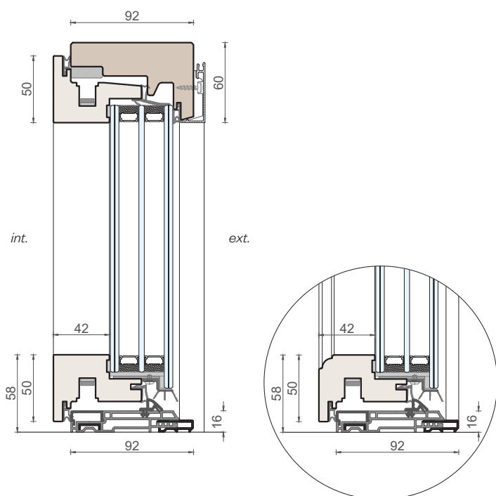
Sezione verticale
