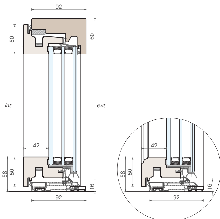
Sezione verticale
