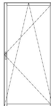
Prospetto
