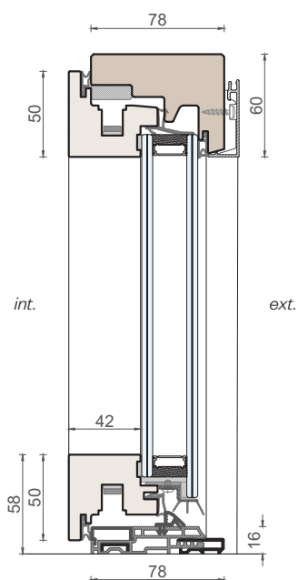
Sezione verticale
