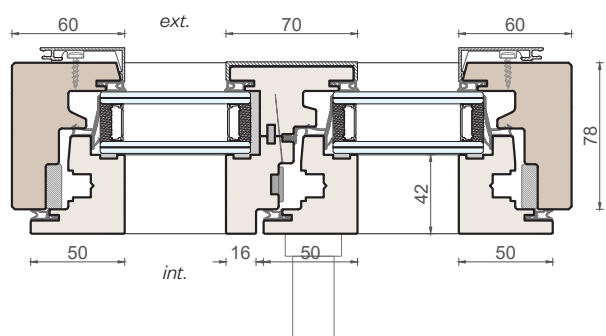
Sezione verticale
