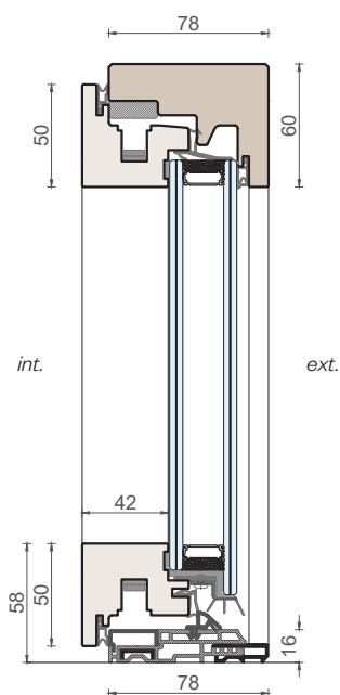
Sezione verticale
